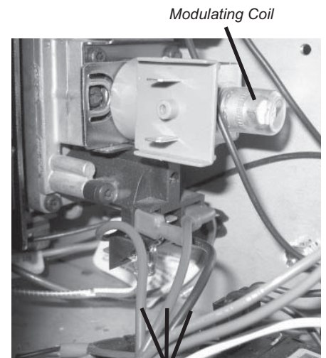
Wires
